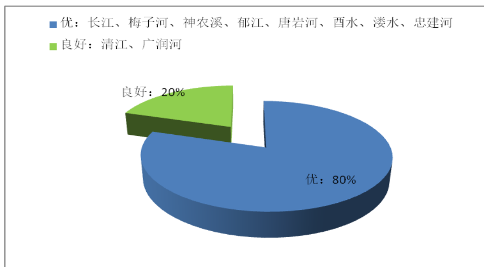
图 1-1 2016年4月恩施自治州主要河流水质优良百分比
