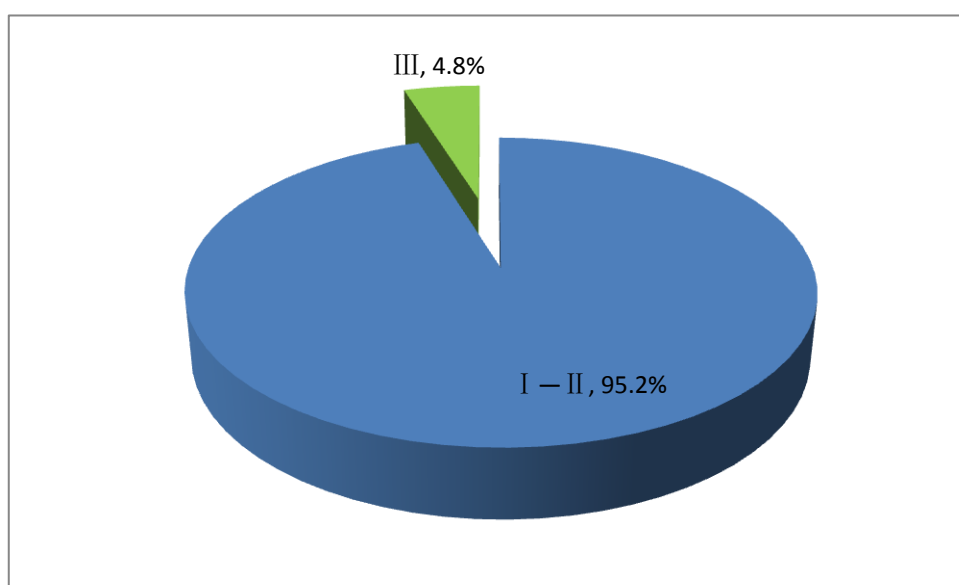
图 1-1 2017 年 11 月主要河流断面水质类别构成比
