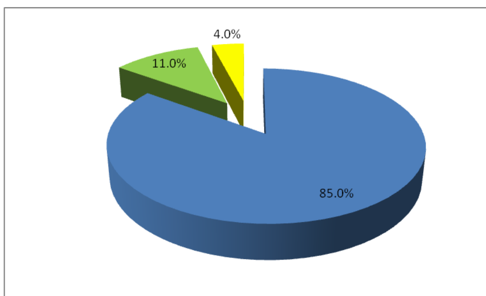
图 1-1 2019年1月主要河流断面水质类别构成比
