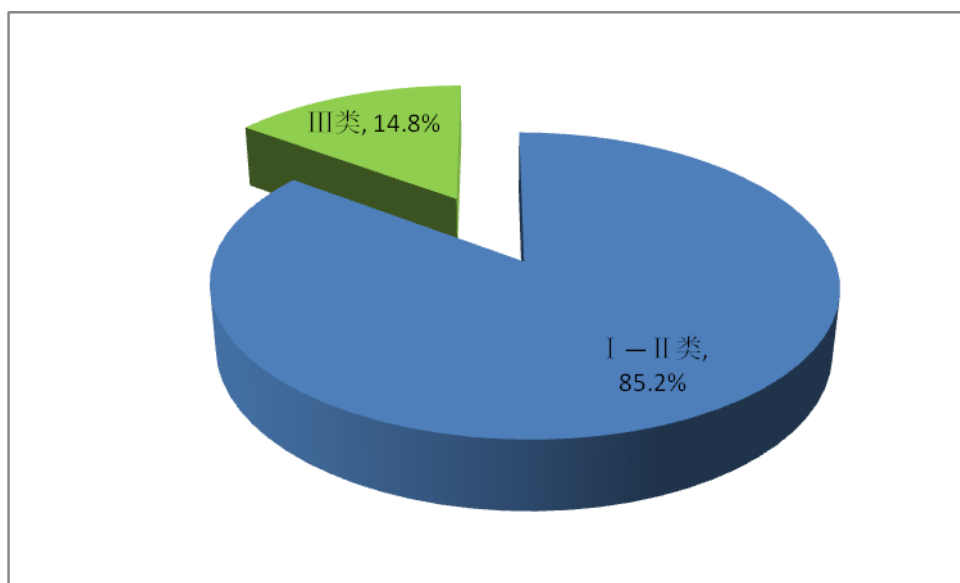
图 1-1 2019年5月主要河流断面水质类别构成比
