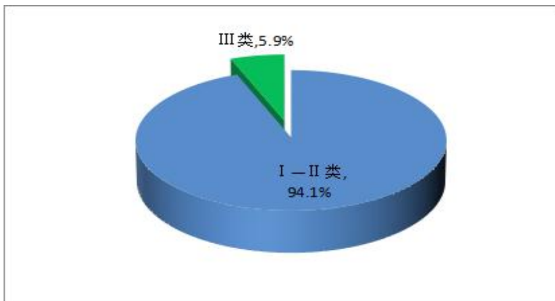
图1 2021年9月主要河流断面水质类别构成比
